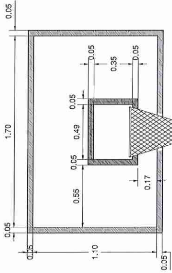
DETALLE DE TABLERO SIN ESCALA
