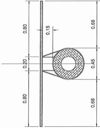
DETALLE DE ARO EN PLANTA SIN ESCALA
