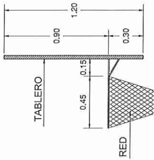
ELEVACIÓN LATERAL DE ARO SIN ESCALA
